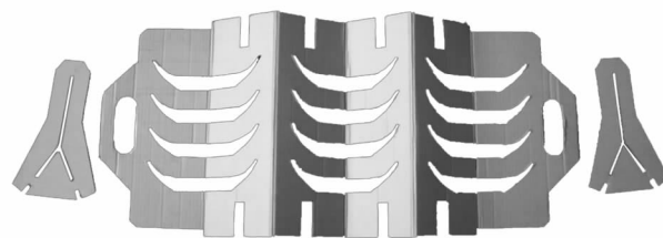
图7 瓷碟包装内衬结构展开图
